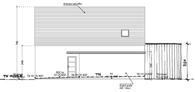
Façade NORD
