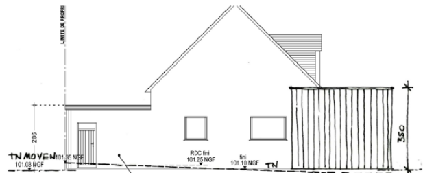
Façade OUEST
