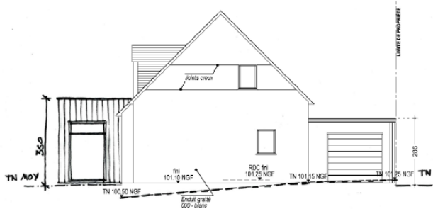
Façade EST
